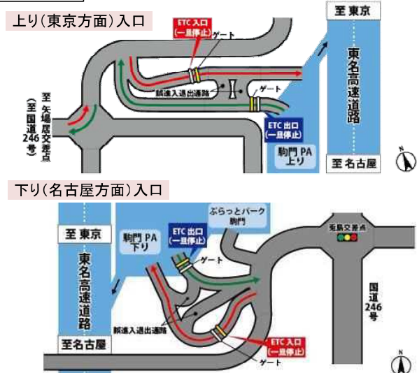
詳細図
